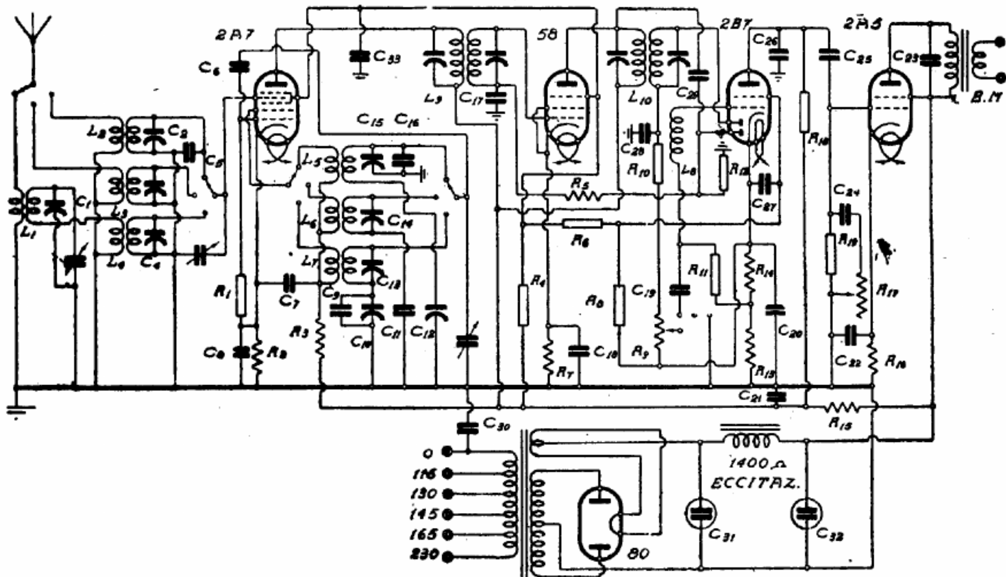
CRESA RADIO - MOD. «SUPERLA 54 CML»
